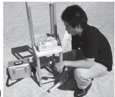
高精度の放射線量測定器で市内52カ所を測定しています
