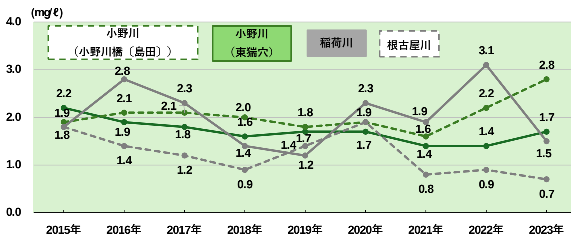
牛久市内の河川の生物化学的酸素要求量（BOD）75%値の経年変化
