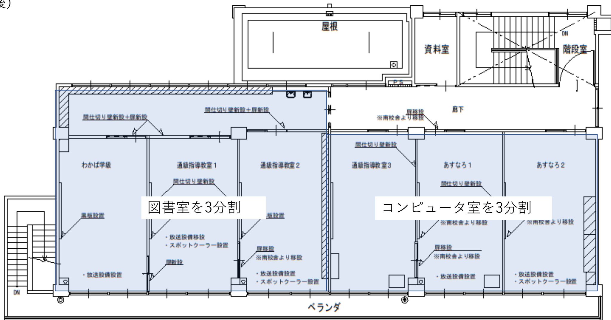
新館3階平面図 (改修後)
