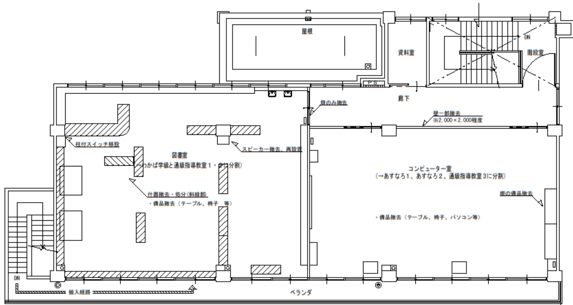
新館 3 階平面図 (既存) 撤去範囲図
