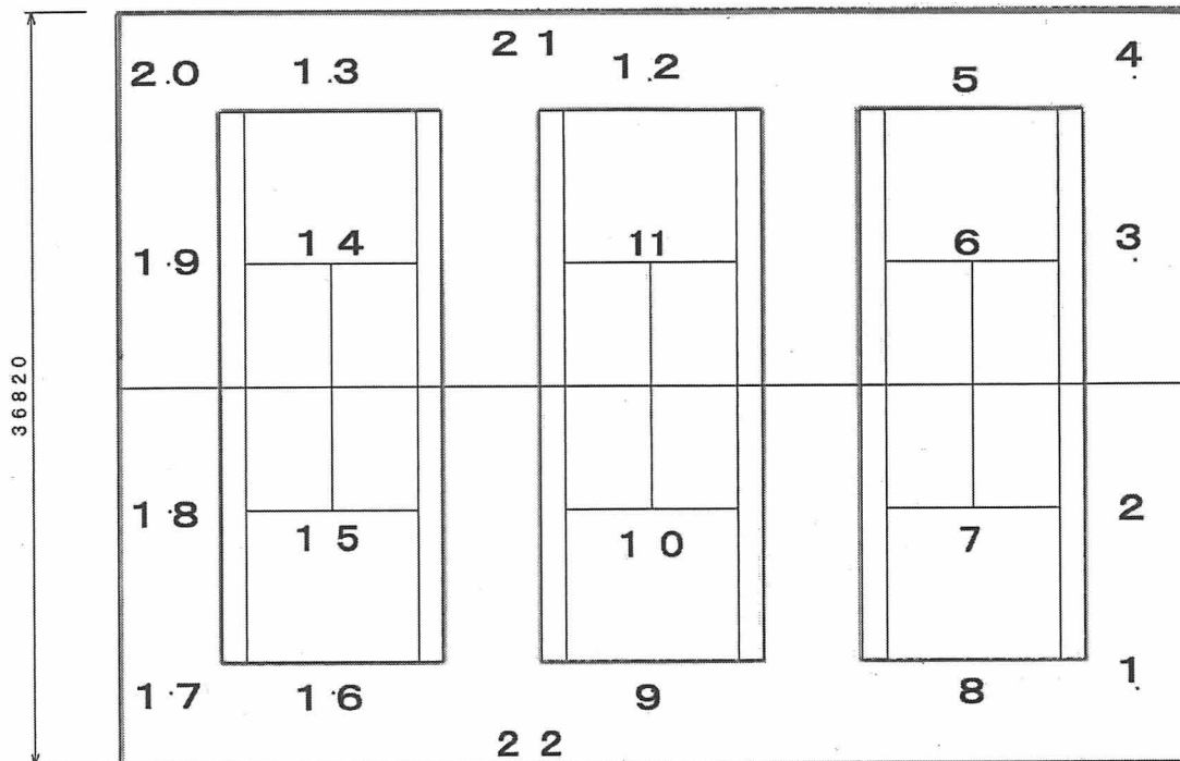
測定位置図
