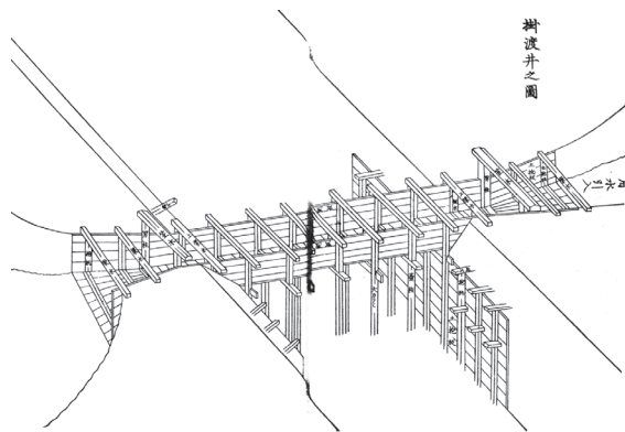
掛渡樋(掛渡井、縣樋ともいう)の図 —土木工要録より引用掲載—
